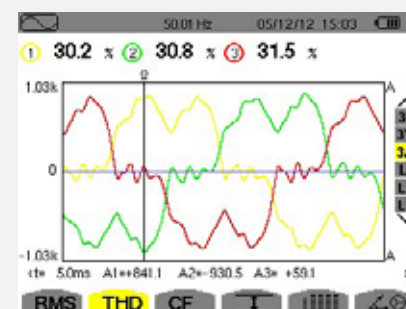
Rete SENZA Econelec+
