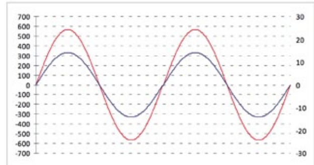
Cos Phi=1
