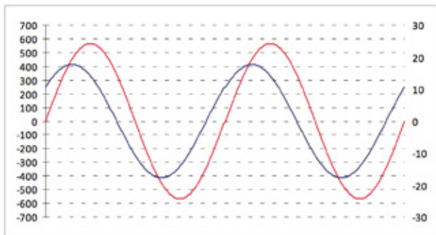
Cos Phi=0,8
