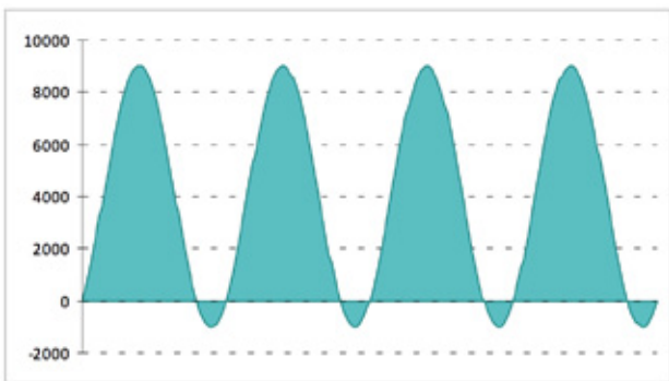
S=5 kVA, P=4kW
